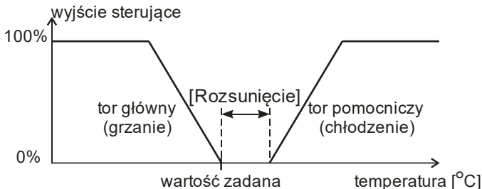
Rys. 22. Regulacja z dwoma torami - typu grzanie-chłodzenie
