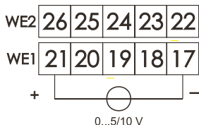
wejście napięciowe 0...5/10 V
