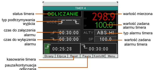
Rys.9. Ekran alarmu pojedynczego timera
