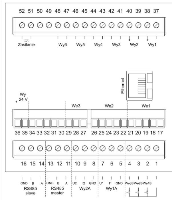
Rys. 3. Widok listew podłączeniowych regulatora.
