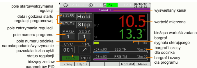
Rys. 7. Ekran z regulacją programową
