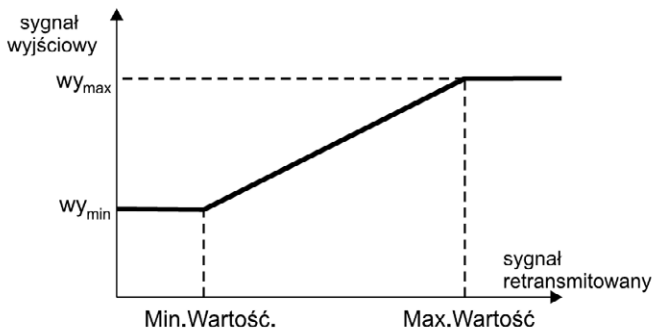
Rys. 21. Przeliczenie sygnału do retransmisji
